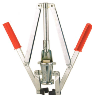
200020 Tappatrice a 2 leve "Vesuvio" per tappi in sughero Ø 2,4 cm., altezza 3,3 cm Ø 2,4 cm., altezza 3,8 cm. (Non è possibile utilizzare tappi di Ø 2,6 cm.)
