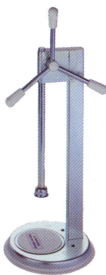
010195 Tappatrice da banco per tappi a corona, a 3 bracci colonna e basamento in ferro verniciato
